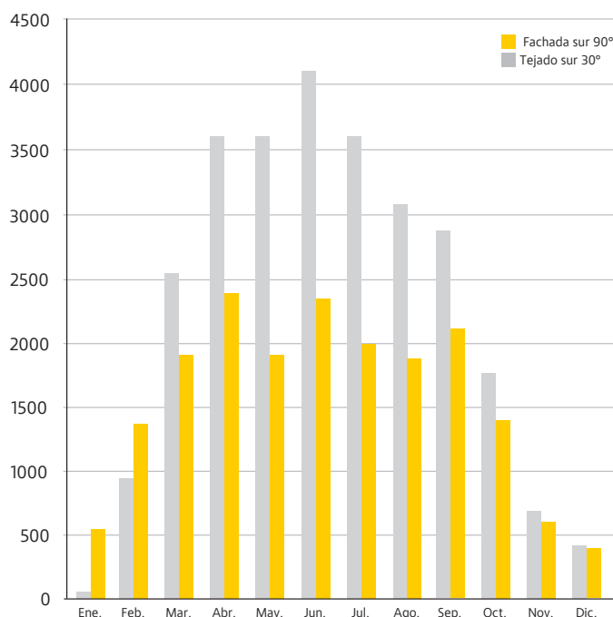
Comparativa de la generación de energía fachada/tejado con un sistema de 30 kWp
