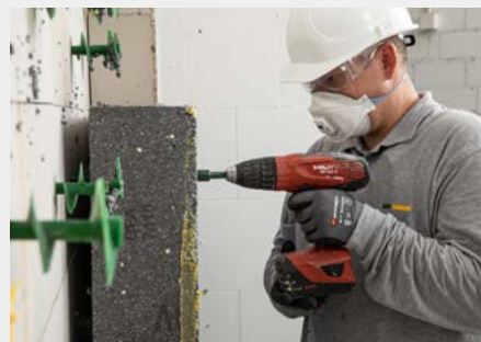
A. Sistemas con fijación mecánica 3. Desmontaje de aislamiento
