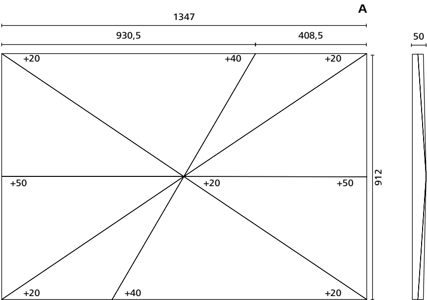
Todas las medidas en mm
