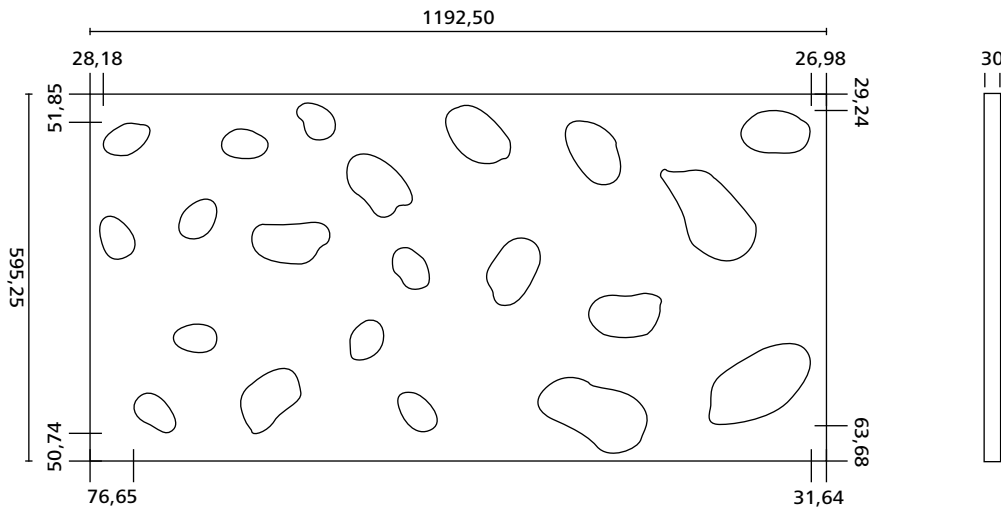
Todas las medidas en mm
