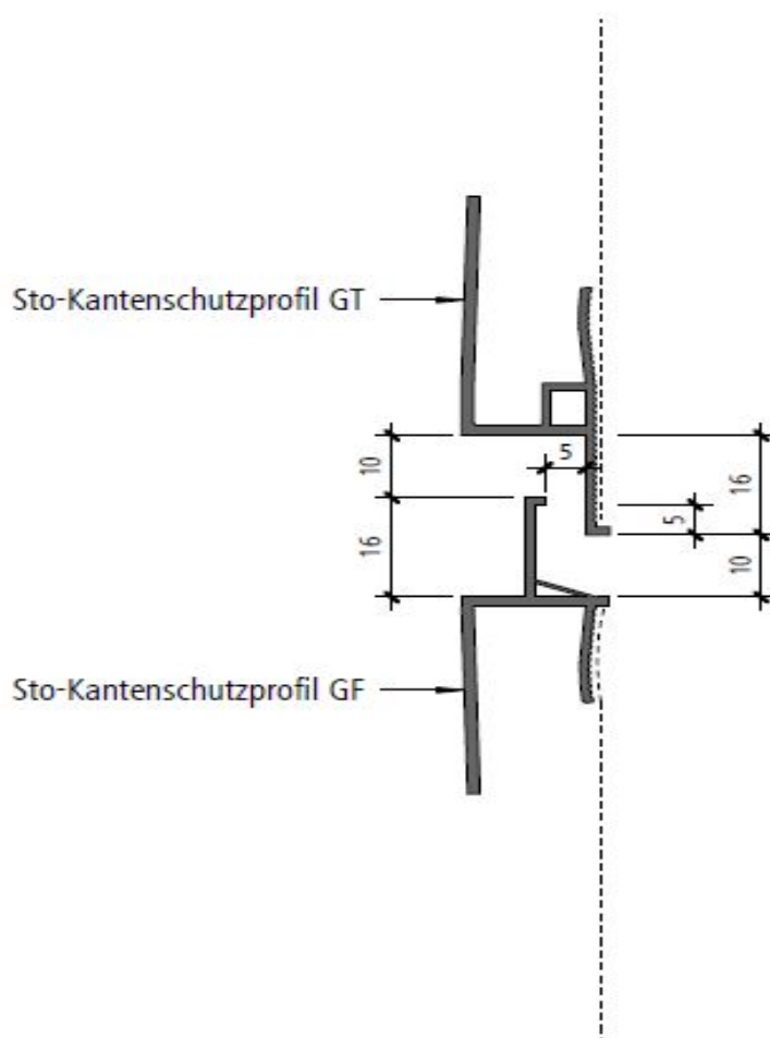
aplicação StoProfile Edge GT/GF
